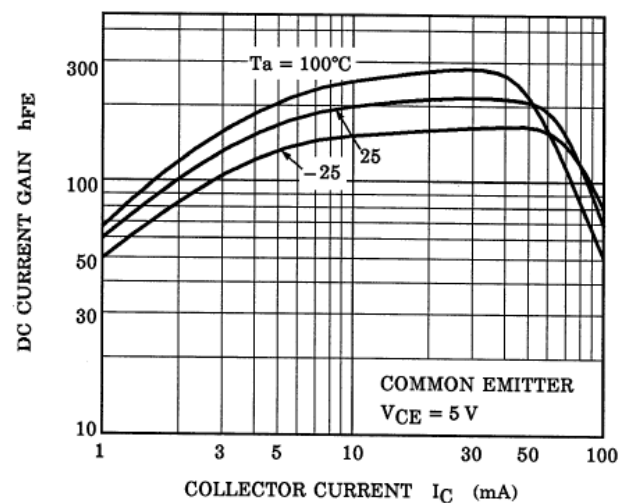
Fig. 10.18 RN1906FE h_{FE} - I_C
