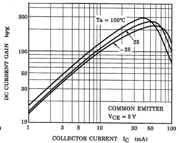
Fig. 10.14 RN1902FE h_{FE} - I_C
