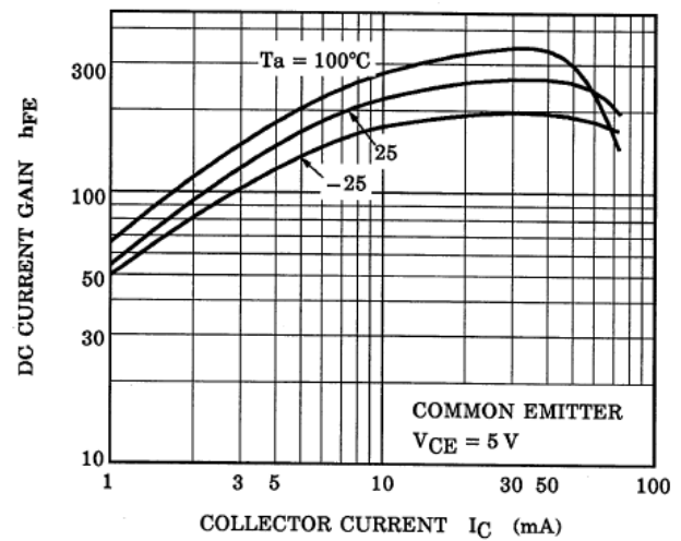
Fig. 10.16 RN1904FE h_{FE} - I_C
