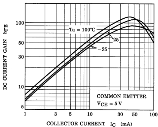
Fig. 10.13 RN1901FE h_{FE} - I_C
