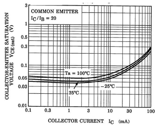
Fig. 9.8 RN1413 V_{CE(sat)}-I_C
