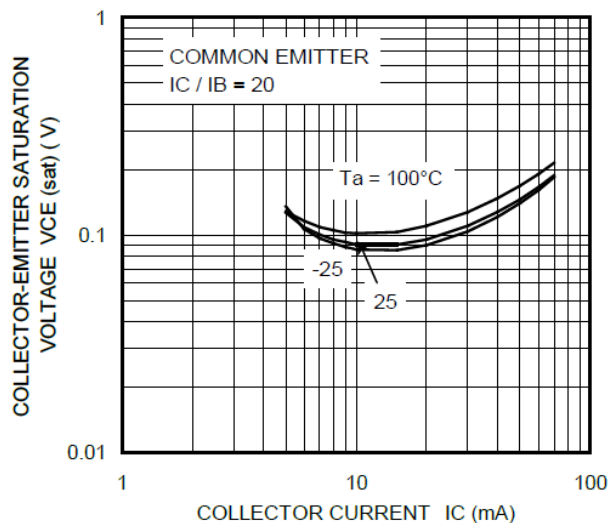
Fig. 10.19 RN1317 V_{CE(sat)}-I_C
