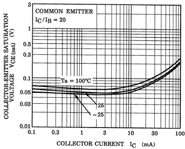
Fig. 9.7 RN1110 V_{CE(sat)}-I_C
