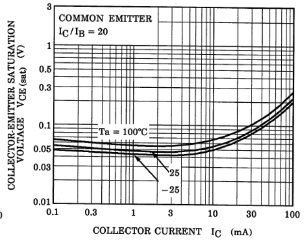
Fig. 9.8 RN1111 V_{CE(sat)}-I_C
