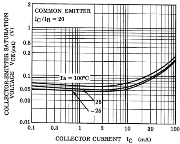
Fig. 9.7 RN1110 V_{CE(sat)}-I_C
