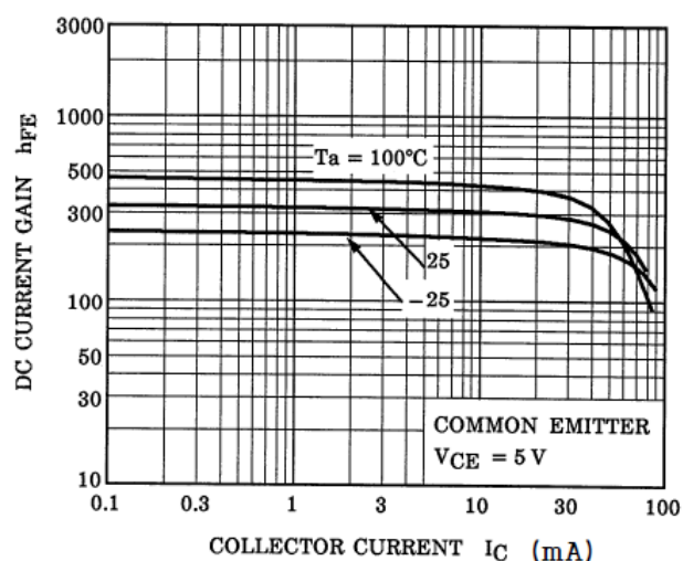
Fig. 9.6 RN1111 h_{FE} - I_C
