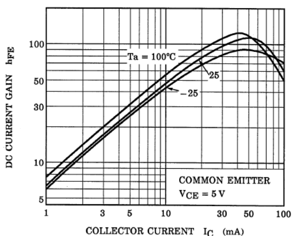
Fig. 10.13 RN1101 h_{FE} - I_C
