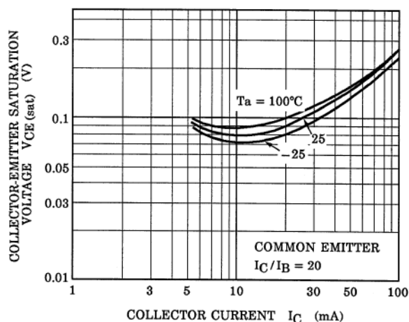
Fig. 10.19 RN1101 V_{CE(sat)}-I_C
