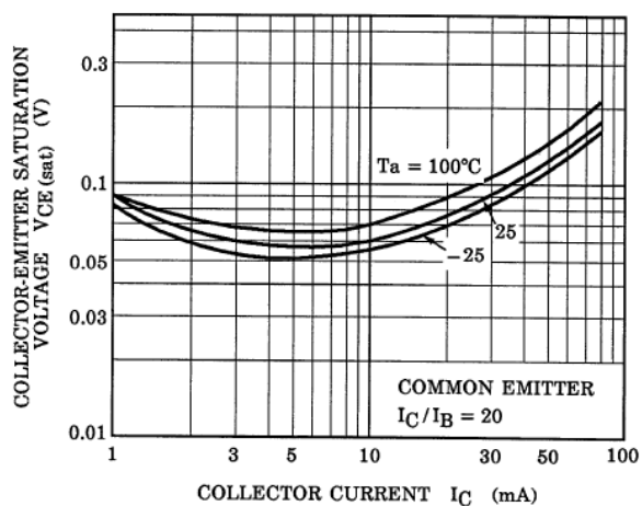
Fig. 10.21 RN1103 V_{CE(sat)}-I_C
