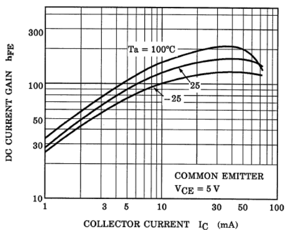
Fig. 10.15 RN1103 h_{FE} - I_C
