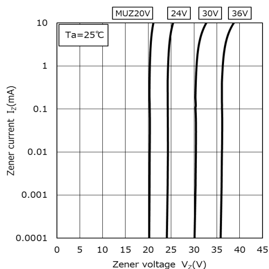
I_Z - V_Z (2)
