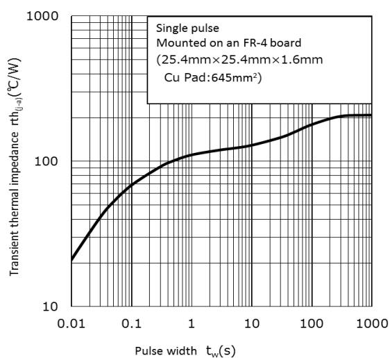
r_{th(j-a)} - t_w
