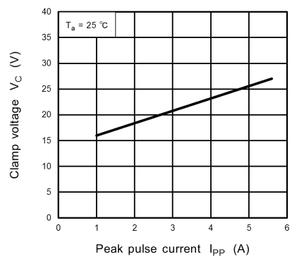
Fig. 10.12.2 V_C - I_{PP}
