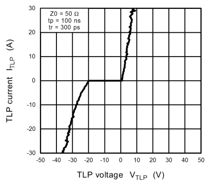
Fig. 10.15.1 I_{TLP} - V_{TLP}
