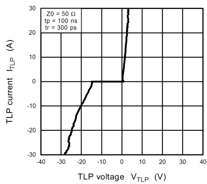
Fig. 10.12.1 I_{TLP} - V_{TLP}
