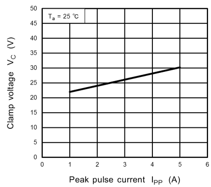
Fig. 10.15.2 V_C - I_{PP}
