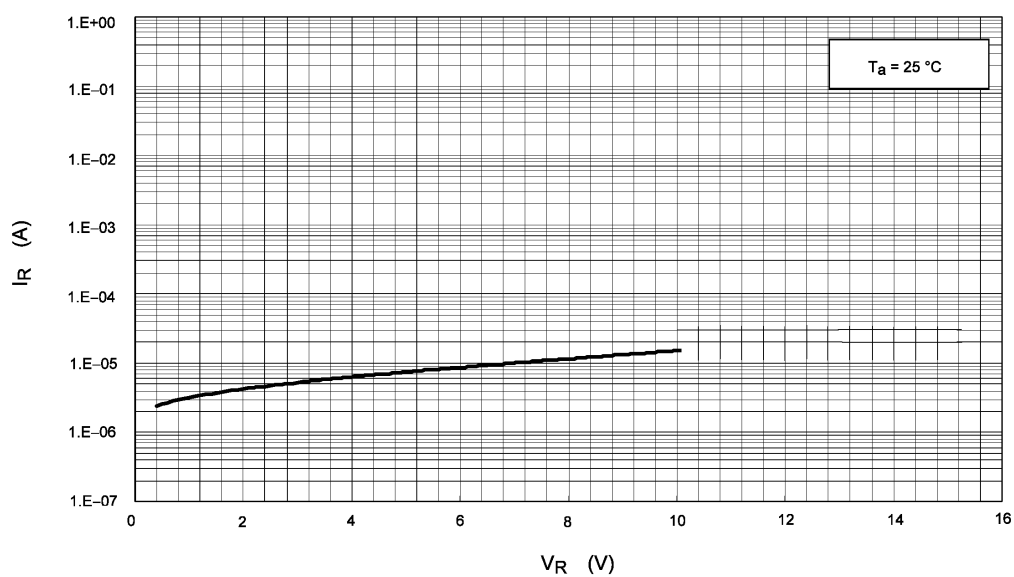
Fig. 9.2 I_R - V_R
