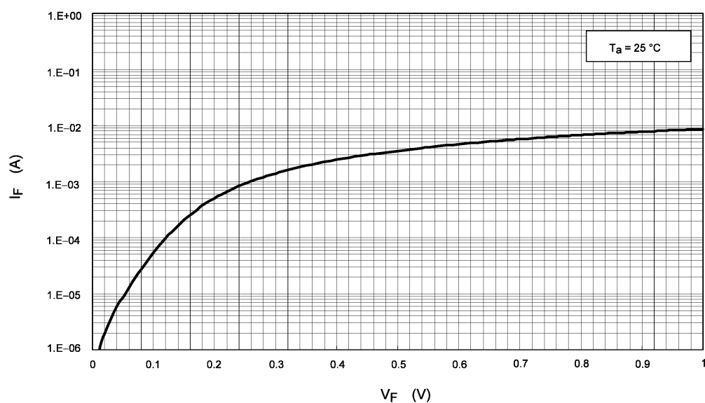
Fig. 9.1 I_F - V_F
