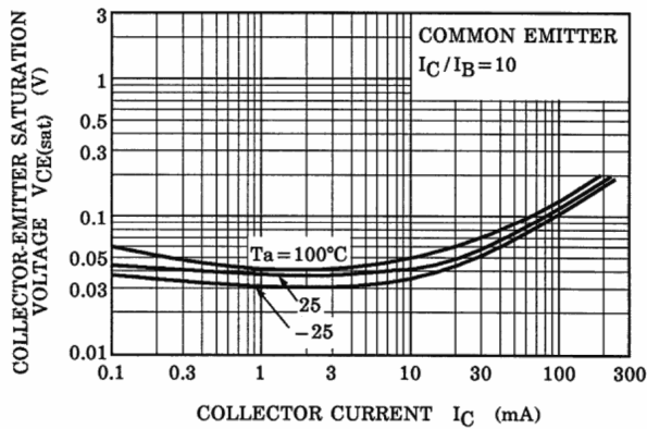
Fig. 14.3 V_{CE(sat)} - I_C
