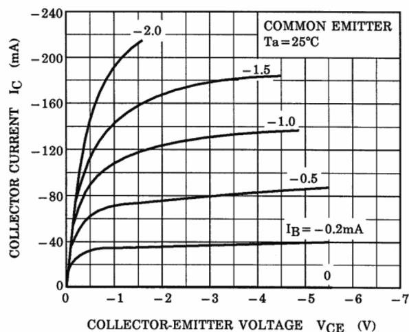
Fig. 13.1 I_C - V_{CE}
