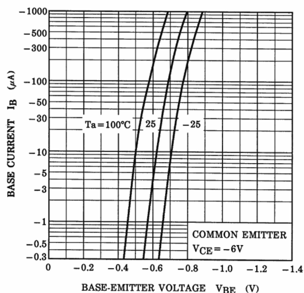
Fig. 13.6 I_B - V_{BE}
