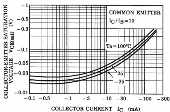
Fig. 13.3 V_{CE(sat)} - I_C
