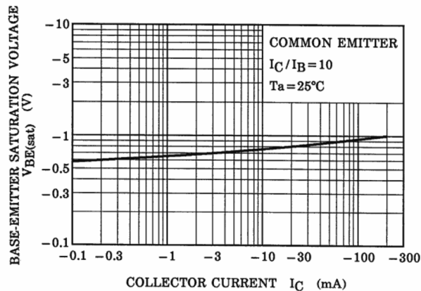
Fig. 13.4 V_{BE(sat)} - I_C
