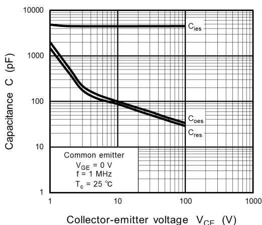
Fig. 8.11 C - V_{CE}
