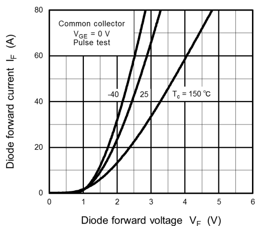
Fig. 8.12 I_F - V_F
