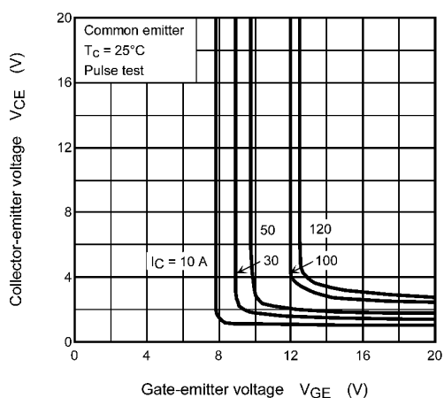
Fig. 8.5 V_{CE} - V_{GE}
