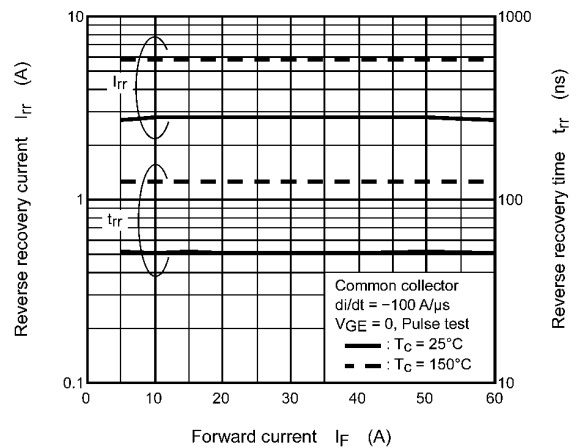
Fig. 8.18 I_{rr} , t_{rr} - I_F
