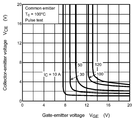
Fig. 8.7 V_{CE} - V_{GE}
