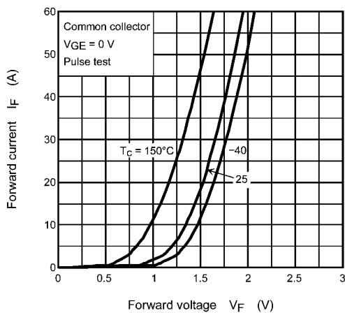
Fig. 8.17 I_F - V_F
