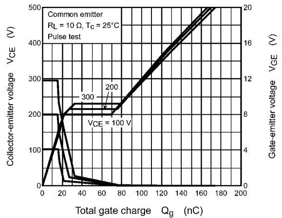
Fig. 8.16 V_{CE} , V_{GE} - Q_g
