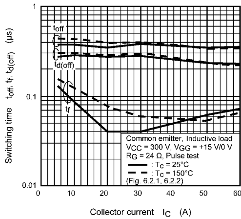
Fig. 8.13 t_{off} , t_r , t_d(off) - I_C
