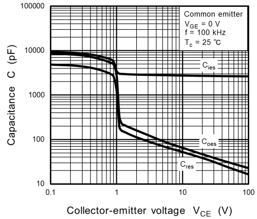
Fig. 8.8 C - V_{CE}
