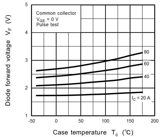
Fig. 8.12 V_F - T_c
