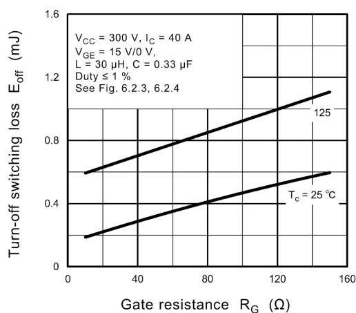
Fig. 8.16 E_{off} - R_G
