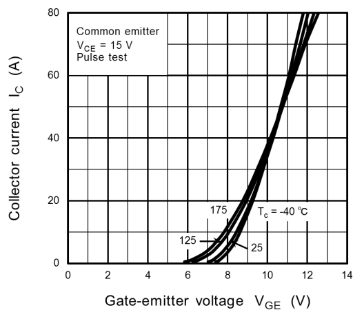
Fig. 8.6 I_C - V_{GE}
