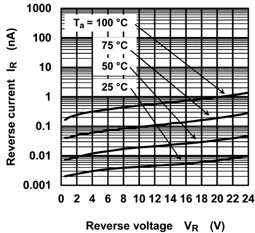
Fig. 9.2 I_R - V_R
