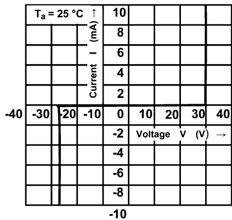
Fig. 9.1 I - V
