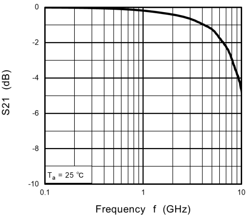
Fig. 9.4 S21 - f
