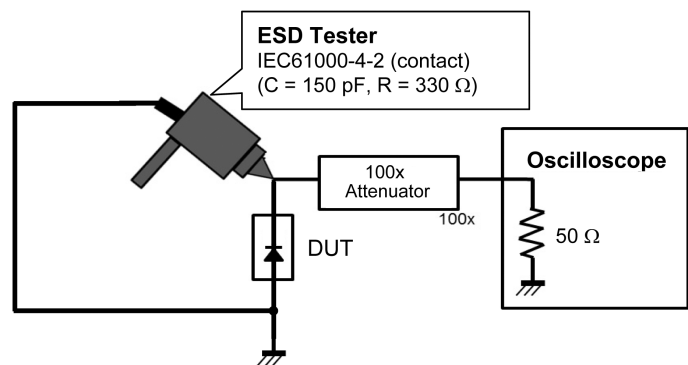
Fig. 6.1.3 IEC61000-4-2 (Contact)
