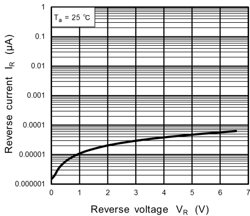
Fig. 9.2 I_R - V_R
