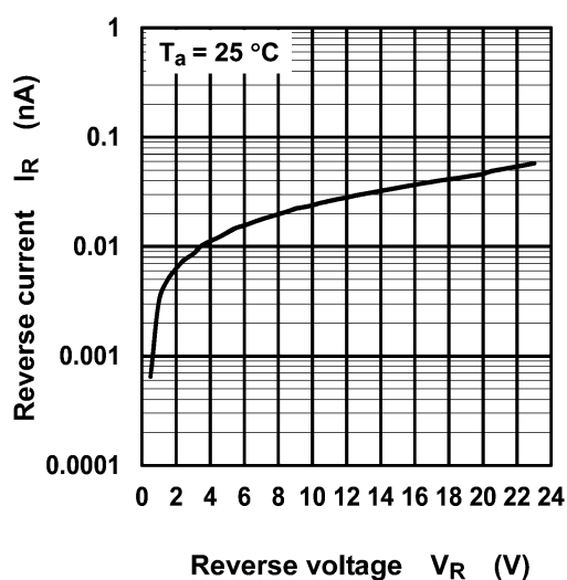
Fig. 8.2 I_R - V_R
