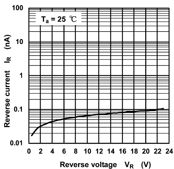
Fig. 8.2 I_R - V_R
