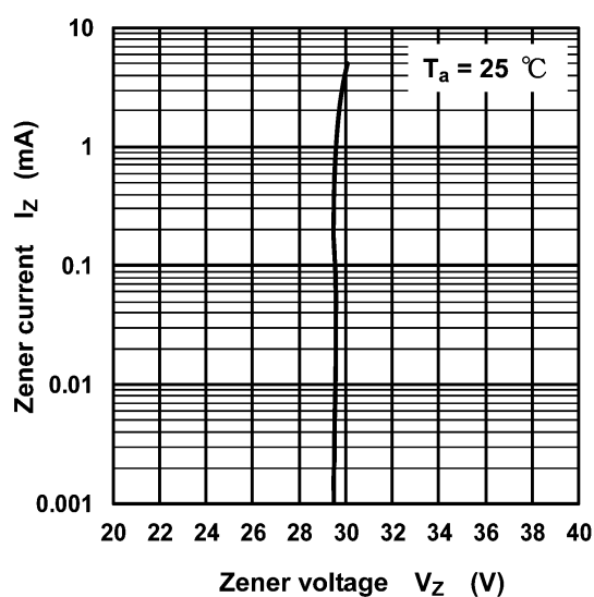
Fig. 8.1 I_Z - V_Z
