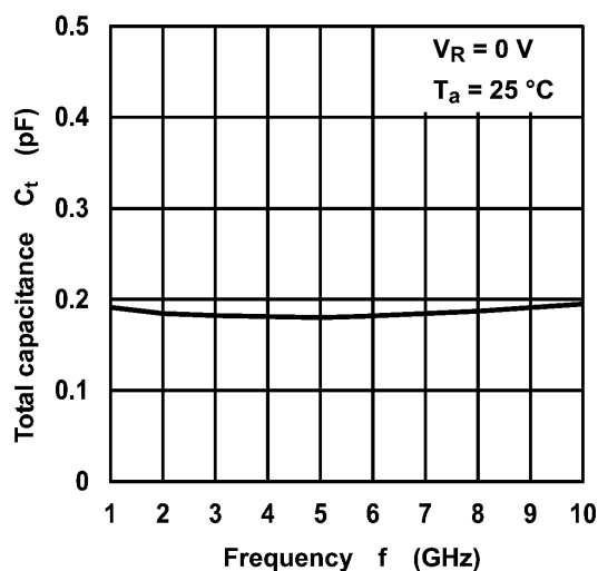
Fig. 7.4 C_t - f
