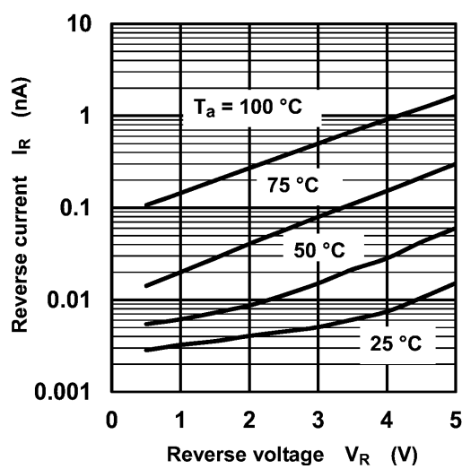
Fig. 7.2 I_R - V_R
