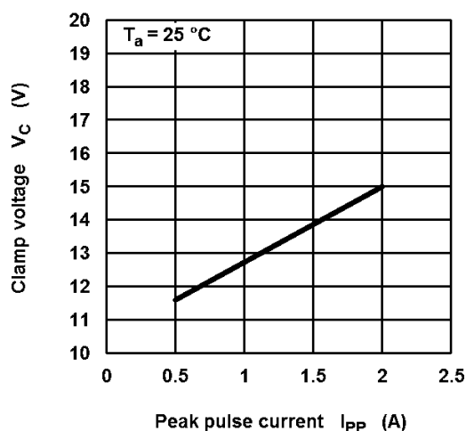
Fig. 8.1 V_C - I_{PP}
