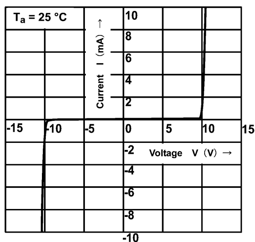
Fig. 7.1 I - V
