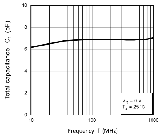
Fig. 8.4 C_t - f
