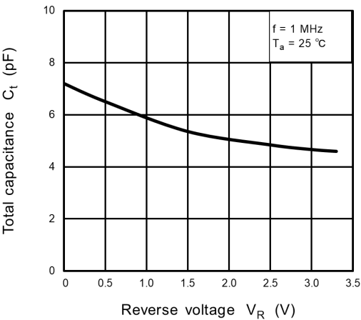
Fig. 9.2 C_t - V_R
