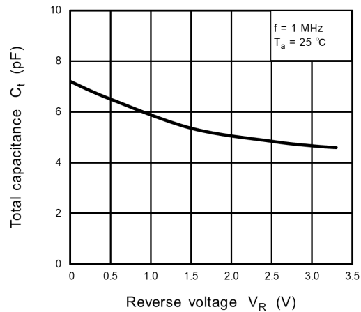
Fig. 9.2 C_t - V_R
