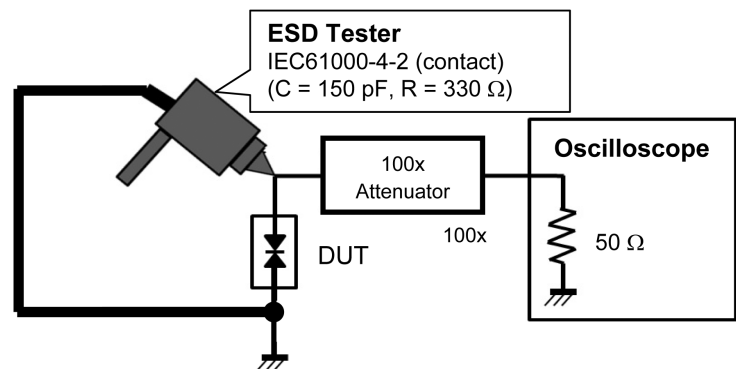
Fig. 6.1.3 IEC61000-4-2 (Contact)
