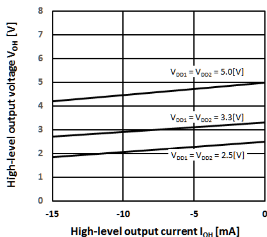
Fig. 13-5: V_{OH} - I_{OH}
