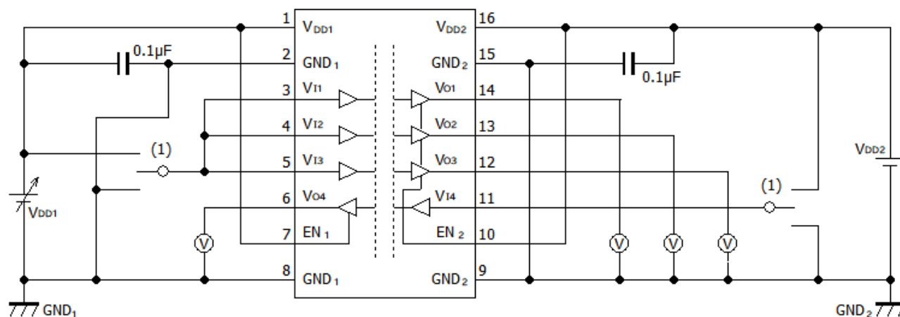
Fig. 12-1: DCL541L01/DCL541H01 V DD1UV+ / V DD1UV- Test Circuit
