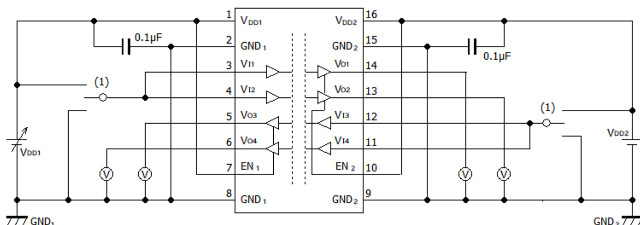
Fig. 12-2: DCL542L01/DCL542H01 V DD1UV+ / V DD1UV- Test Circuit
