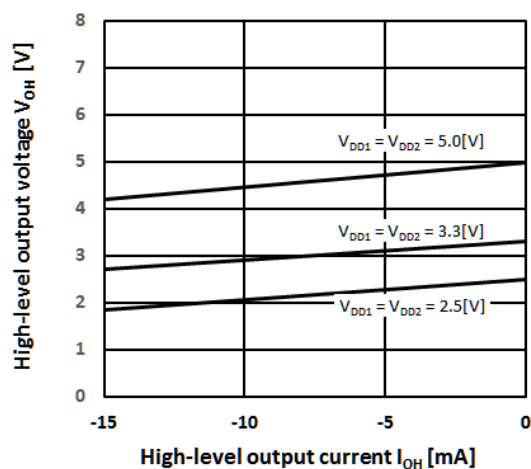
Fig.13-5. V_{OH} - I_{OH}
