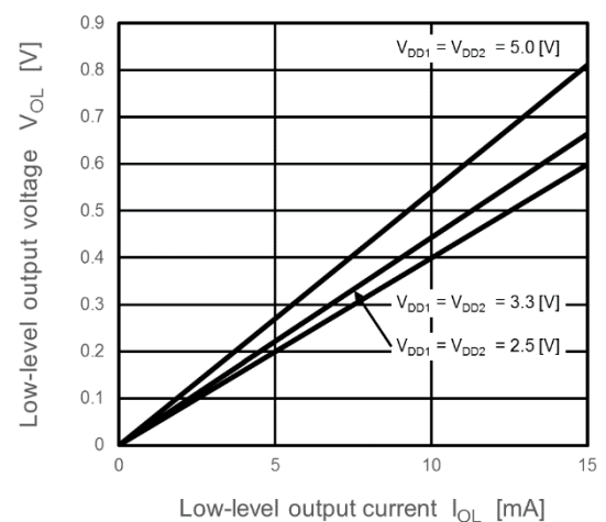
Fig.13-6. V_{OL} - I_{OL}
