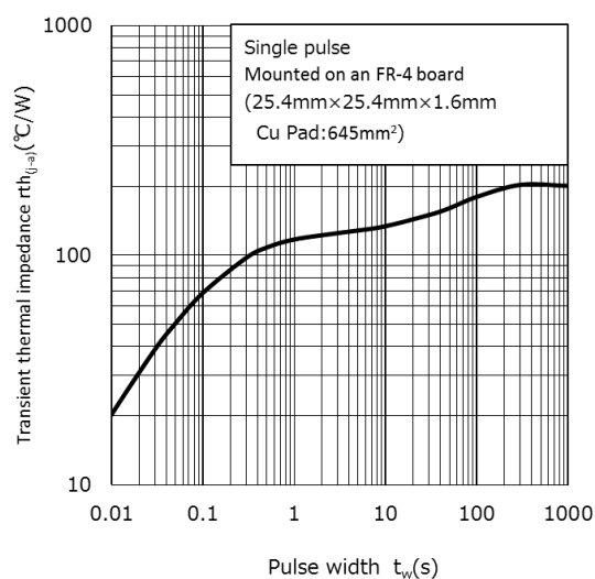
r_{th(j-a)} - t_w
