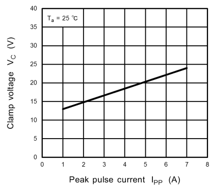
Fig. 10.10.2 V_C - I_{PP}
