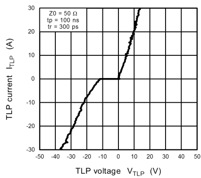
Fig. 10.10.1 I_{TLP} - V_{TLP}
