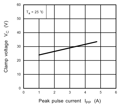
Fig. 10.16.2 V_C - I_{PP}
