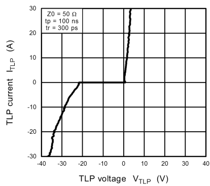
Fig. 10.16.1 I_{TLP} - V_{TLP}
