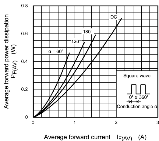
Fig. 10.2 P_{F(AV)} - I_{F(AV)}
