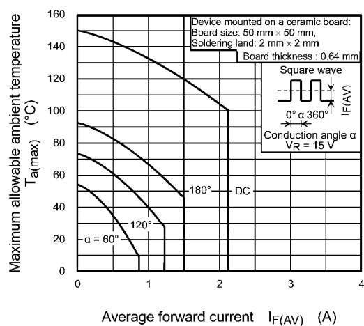
Fig. 10.3 T_{a(max)} - I_{F(AV)}
