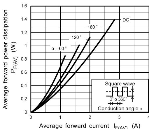
Fig. 10.2 P_{F(AV)} - I_{F(AV)}
