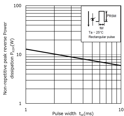
P_{RSM} - t_w
