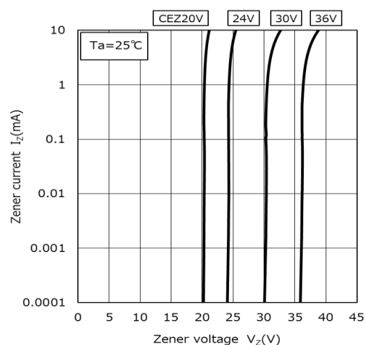
I_Z - V_Z (2)
