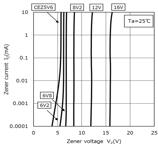
I_Z - V_Z (1)
