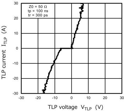
Fig. 10.4.1 I_{TLP} - V_{TLP}
