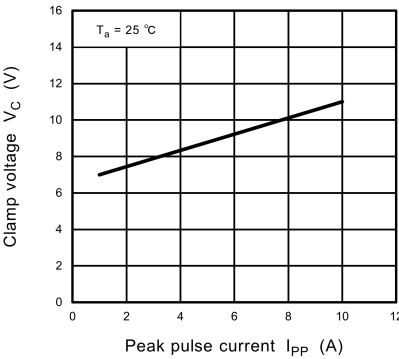
Fig. 10.4.2 V_C - I_{PP}
