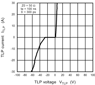
Fig. 10.18.1 I_{TLP} - V_{TLP}
