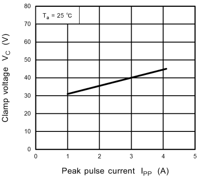
Fig. 10.18.2 V_C - I_{PP}
