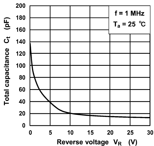
Fig. 8.3 C_t - V_R
