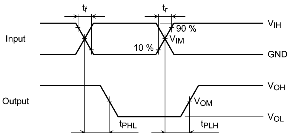
Fig. 11.8.1 t_{PLH}, t_{PHL}
