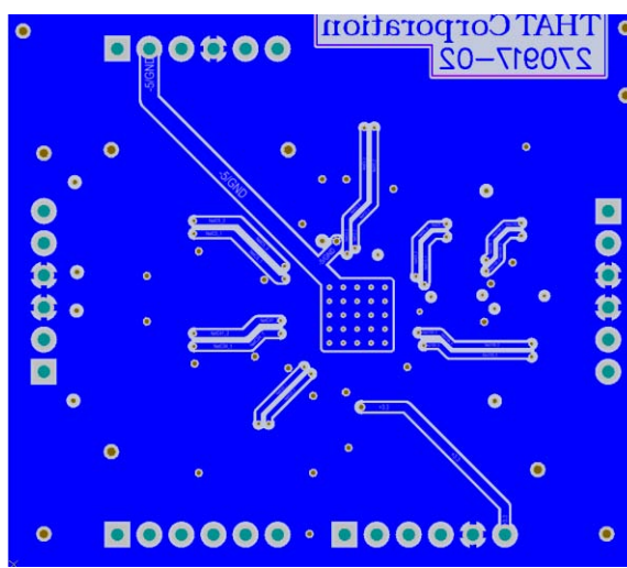
IC Module, Bottom Layer
