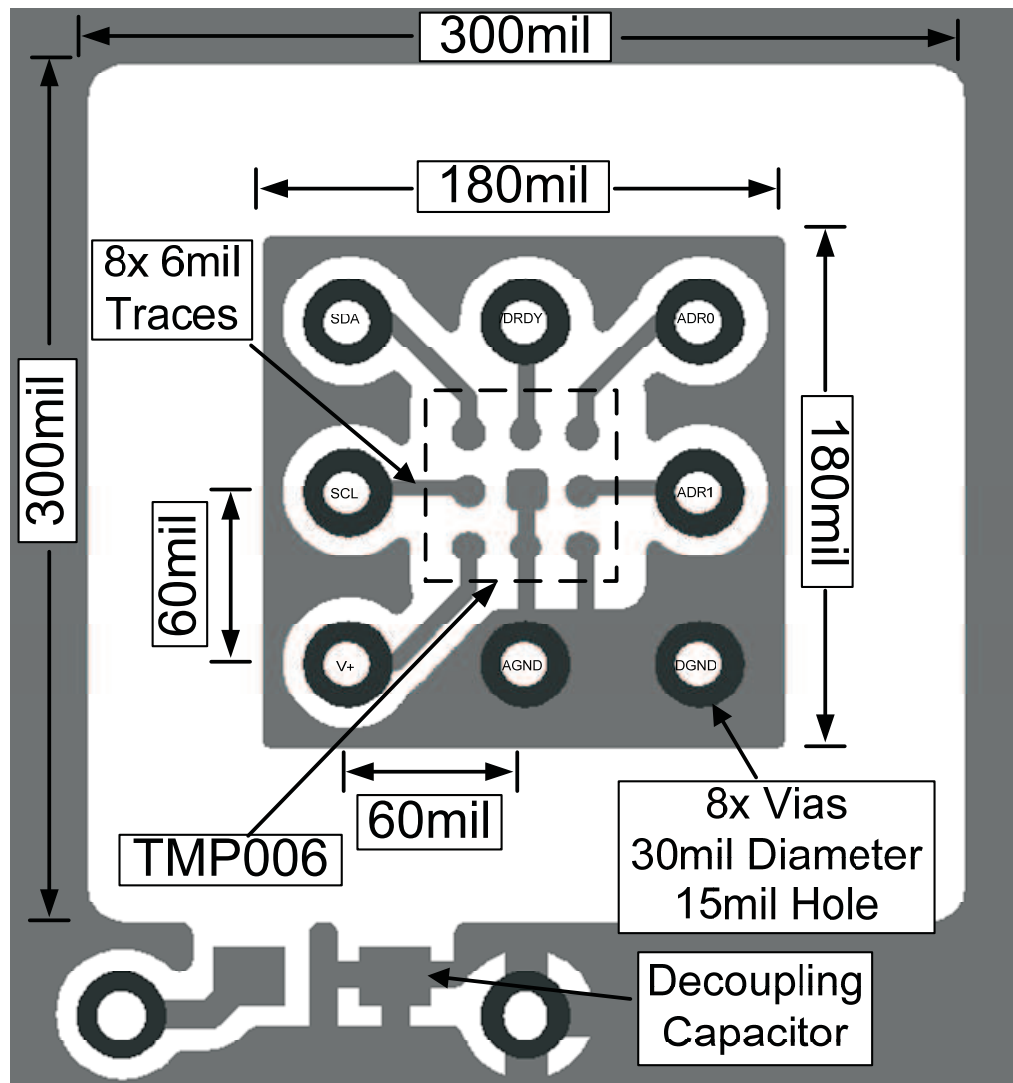
Figure 22. Top Layer
