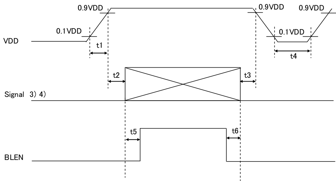
1) V DD -turn-on conditions
