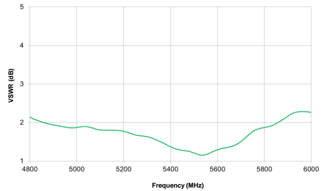
5 GHz VSWR
