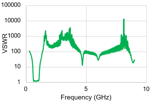
VSWR
