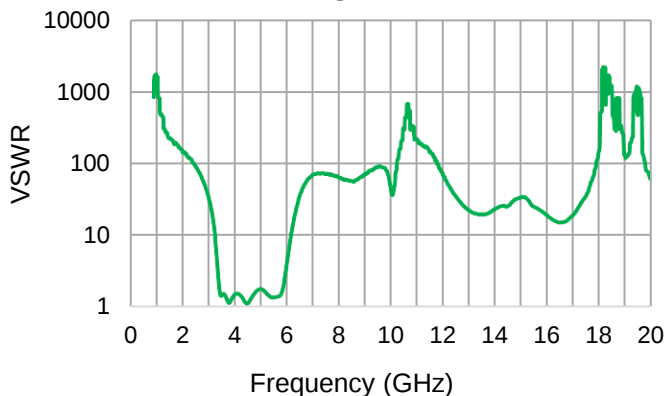
VSWR
