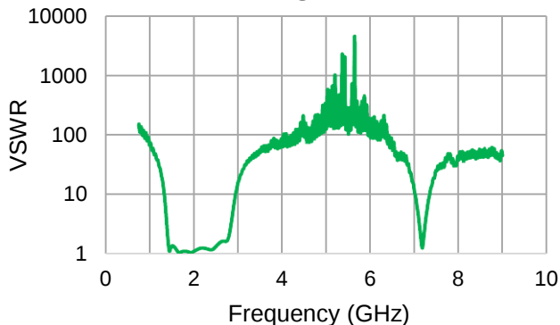
VSWR
