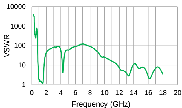
VSWR
