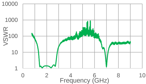
VSWR
