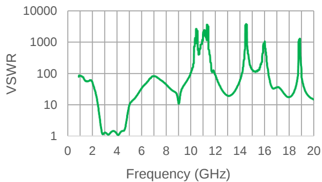
VSWR
