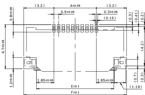
推奨パターン寸法
