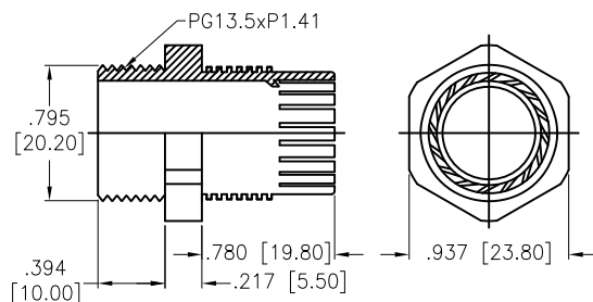
Ⓒ Body
