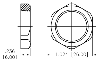
Ⓐ Lock Nut
