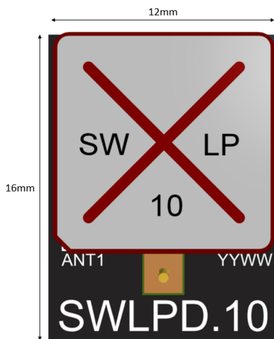
Top Side
